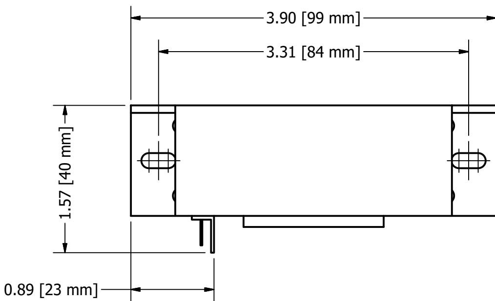
CTI-500 SCALE 1 : 1
